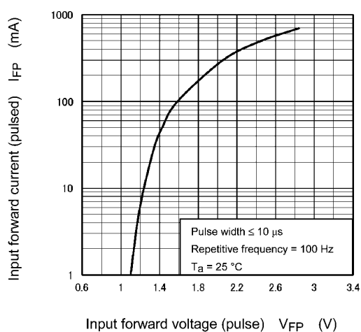
Fig. 11.6 I_{FP} - V_{FP}
