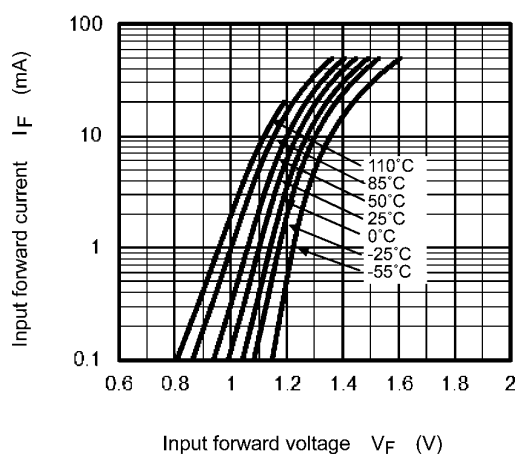
Fig. 11.4 I_F - V_F
