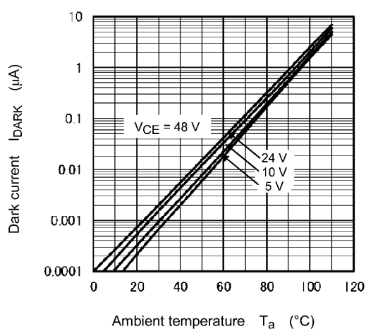
Fig. 11.11 I_{DARK} - T_A
